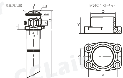
法兰式(出油口法兰连接)
